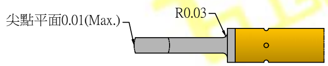
強化結構示意圖
